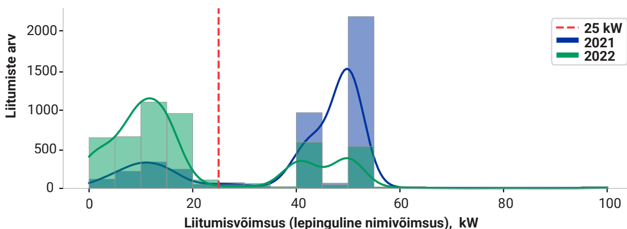
Joonis 8. Elektri võrguga liitunud päikeseparkide arv ja tootmisvõimsused 2021 ja 2022
