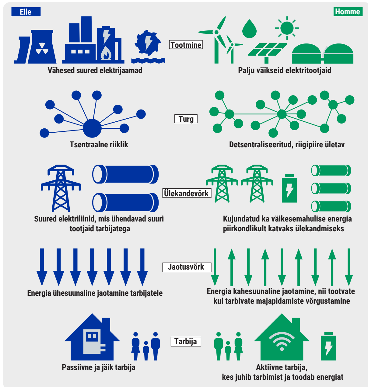
Joonis 1. Elektrisüsteem täna ja homme
