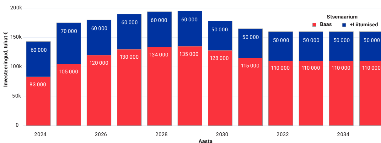
Joonis 32. Jaotusvõrgu investeeringute prognoos aastateks 2024–2035
